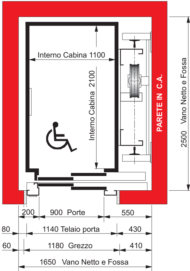
PIANTA VANO CORSA
