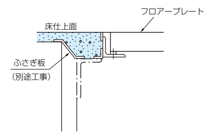
B-B断面
