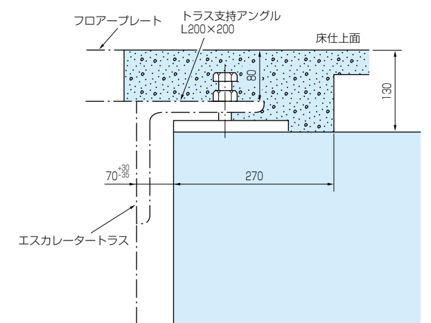
支持梁がコンクリートのとき
