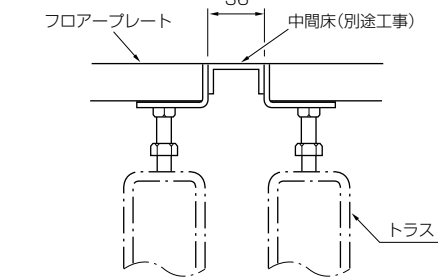
C-C断面
