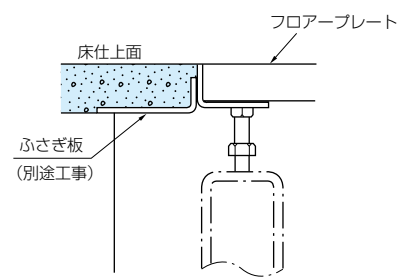
B-B断面
