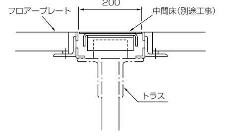
C-C断面
