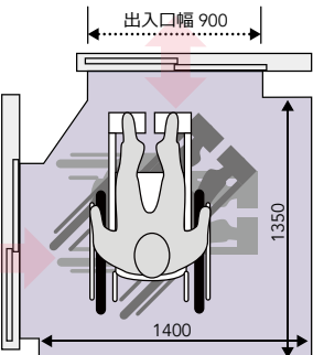
11人乗り 直角二方向出入口 VPL-11B3
