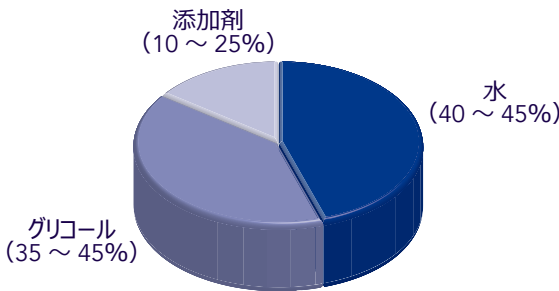
水 - グリコール系作動液の代表的な組成グラフ (設置環境等により異なる)
