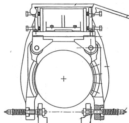
17CT(2005 年 11 月之后产品) 结构示意图
