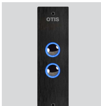
Placca in acciaio inox BLACK hairline, due bottoni in acciaio inox con retroilluminazione blu
