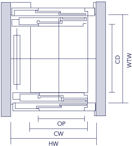
ZWEISEITIGER EINSTIEG
