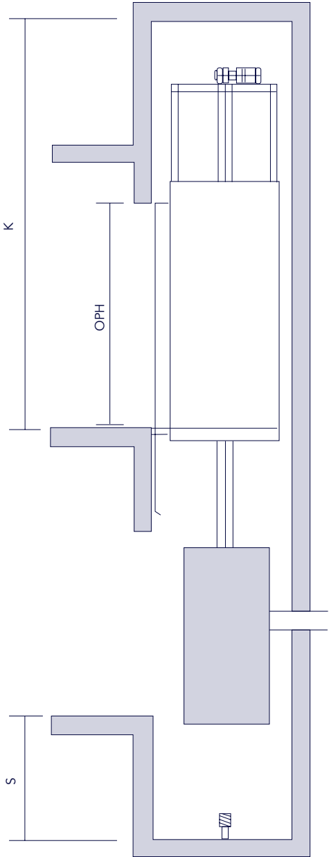
VERTIKALER SCHNITT
