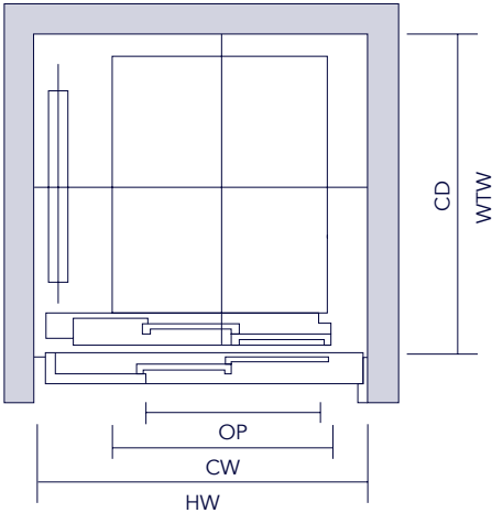
EINSEITIGER EINSTIEG
