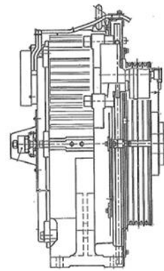
明電製 T3.5/5.2/6.8 (ギヤレスマシン)
