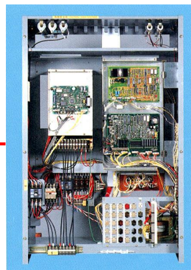
制御盤
