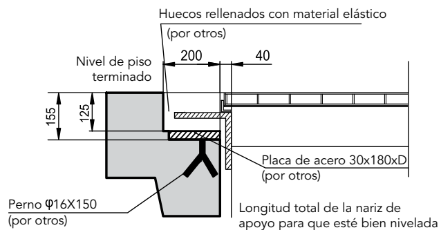
DETALLE DEL SOPORTE U/D (Simetría)
