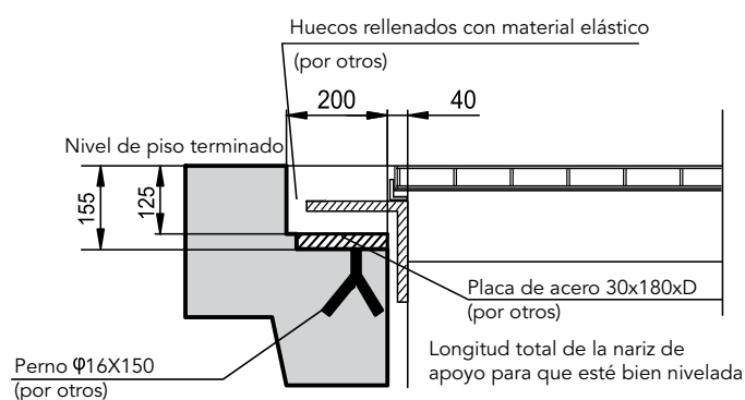
DETALLE DEL APOYO U/D
