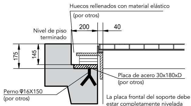
DETALLE DEL SOPORTE U/D (Simetría)
