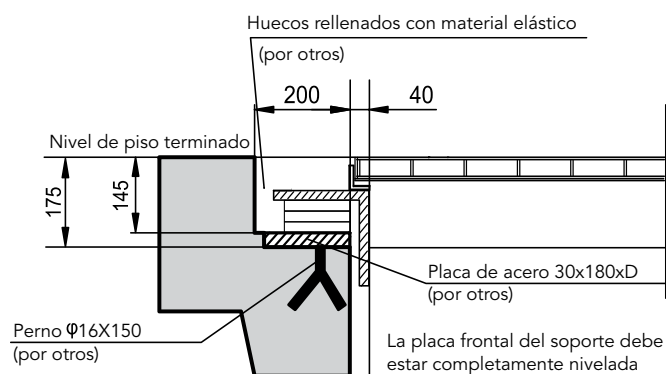
DETALLE DEL SOPORTE U/D (Simetría)
