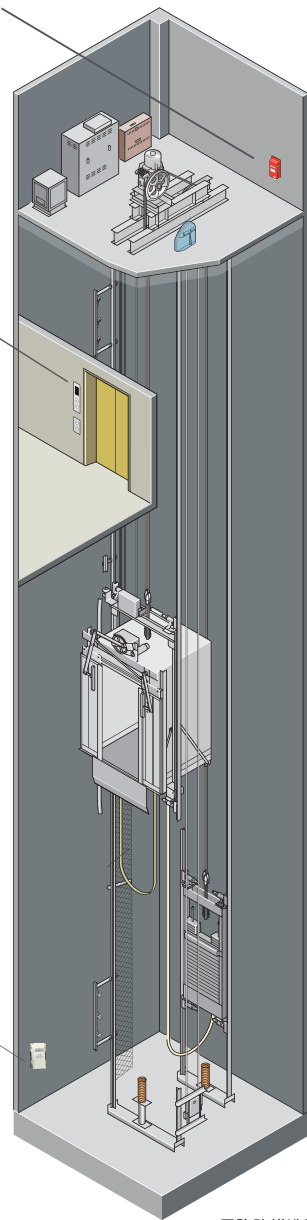
昇降路構造図
