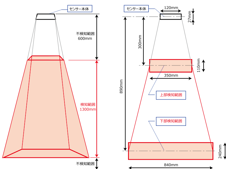
検知範囲（出入口正面）
