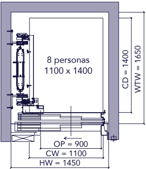
Un embarque, estribo lateral
