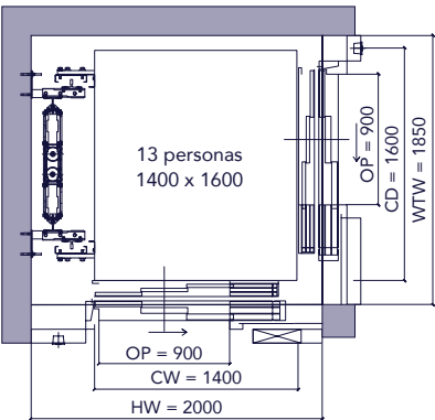
Doble embarque 90°, estribo lateral
