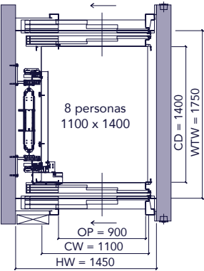
Doble embarque 180°, estribo lateral
